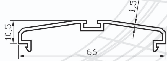
2715 ÇARPMA KAPI ADAPTÖRÜ GENİŞ
