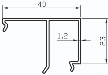
2607 ÇITA 4 mm tek cam için)
