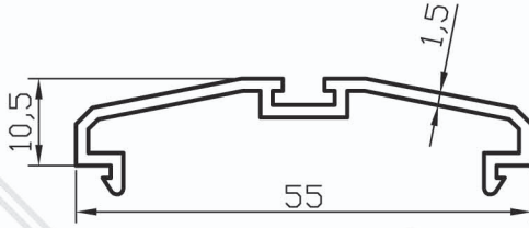
2714 ÇARPMA KAPI ADAPTÖRÜ DAR
