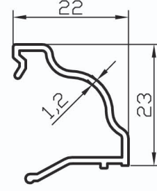
2626 OVAL ÇITA ( 4+12+4 cam için)
