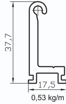
2715 ÇARPMA KAPI ADAPTÖRÜ GENİŞ
