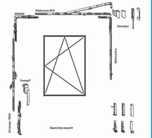
Çift açılım mekanizması
